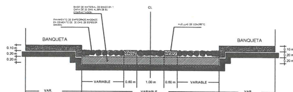
DETALLE CONSTRUCTIVO
