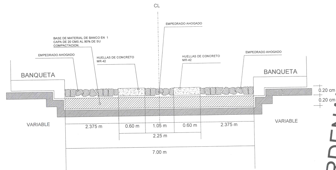
DETALLE CONSTRUCTIVO PROPUESTO
