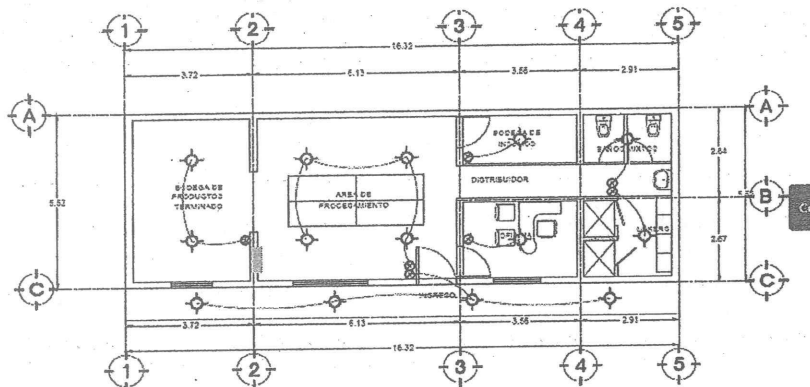
PLANTA INSTALACION ELECTRICA
