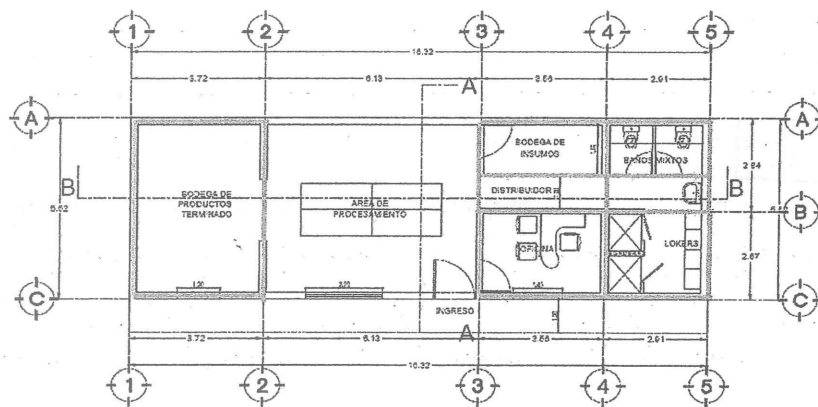
PLANTA ARQUITECTONICA
