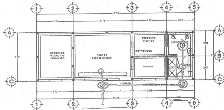
PLANTA DE CIMENTACION Y DRENAJE
