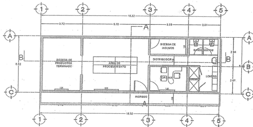
PLANTA ARQUITECTONICA
