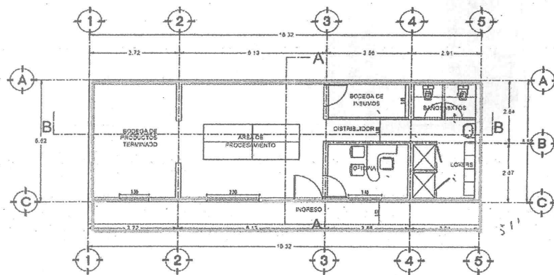
PLANTA ARQUITECTONICA
