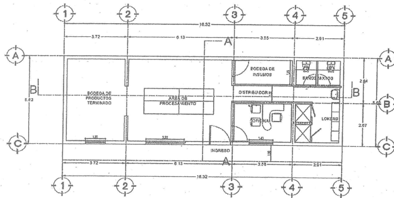
PLANTA ARQUITECTONICA
