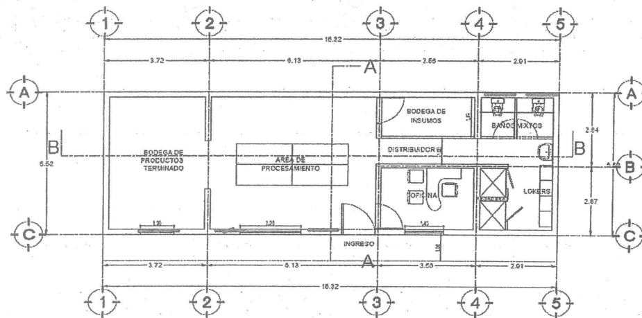
PLANTA ARQUITECTONICA
