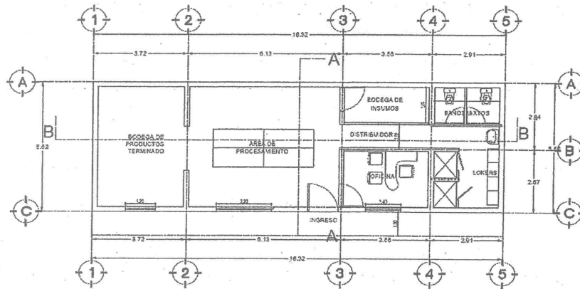
PLANTA ARQUITECTONICA
