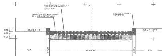
DETALLE CONSTRUCTIVO
